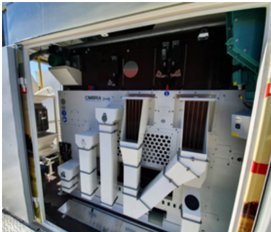
02/ Potrubný magnet a čistička Delta s plochými sitami
